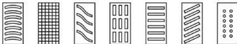
Рисунок 1 — Типовые конструкции водоръемных решеток
