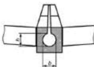
h, b — внутренние размеры (смазываемый периметр)
