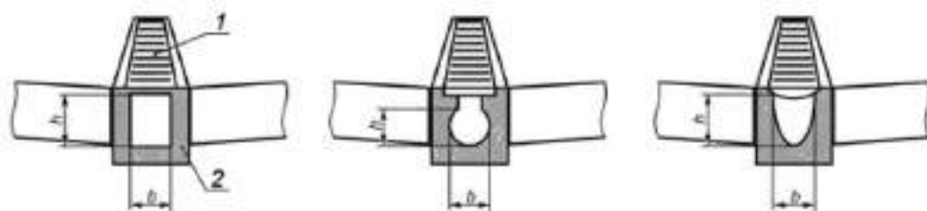
1 — решетка; 2 — корпус лотка; h, b — внутренние размеры (смазываемый периметр)
